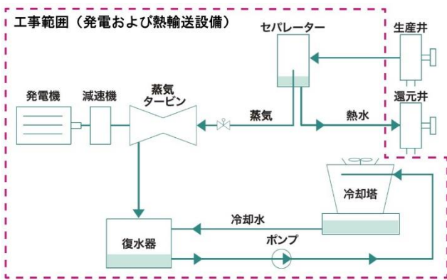
本発電所の仕組みと工事範囲
