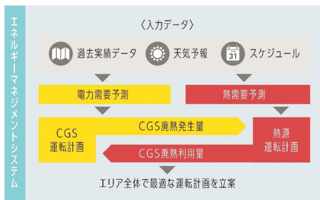
EMS 概念図
