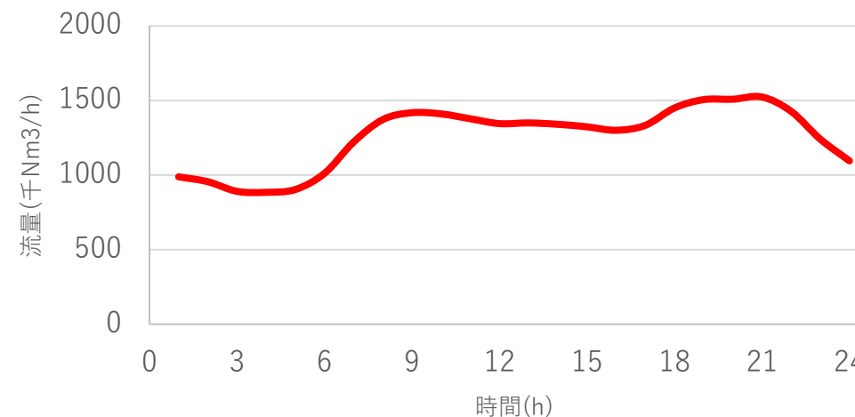
扇島・根岸エリアロードカーブ(ピーク日平均)
