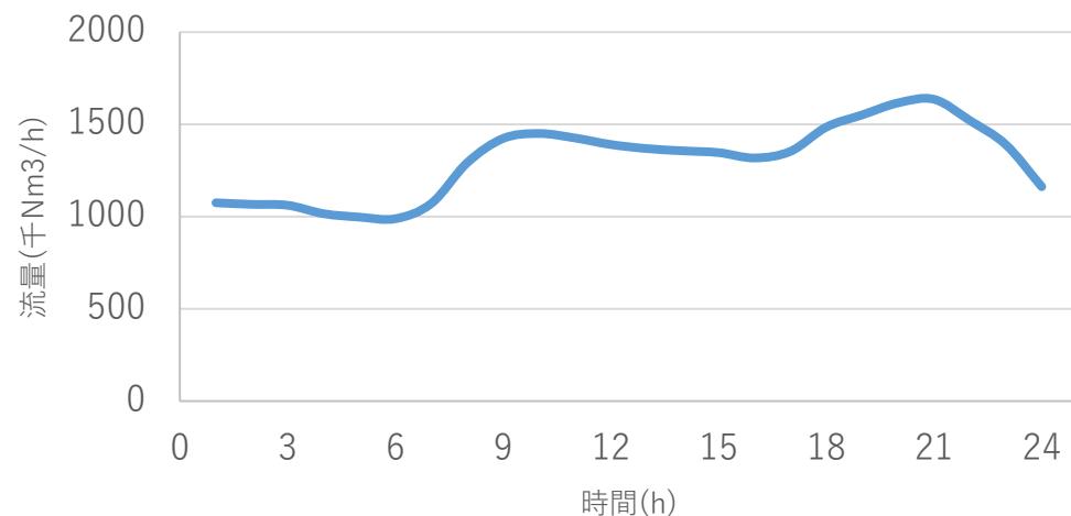
袖ヶ浦・日立エリアロードカーブ(ピーク日平均)
