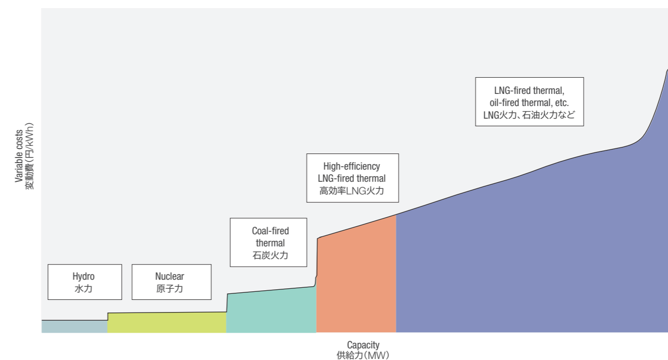
Generation Costs by Power Source in Japan (Variable cost) (image) (Yen/kWh) 日本の各電源の発電コスト(変動費)(イメージ)(円/kWh)
