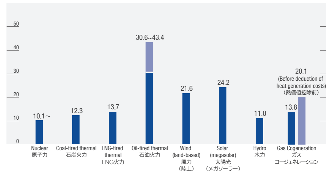
Generation Costs by Power Source in Japan (2014 Model Plants) (Yen/kWh) 日本の各電源の発電コスト(2014年モデルプラント)(円/kWh)
