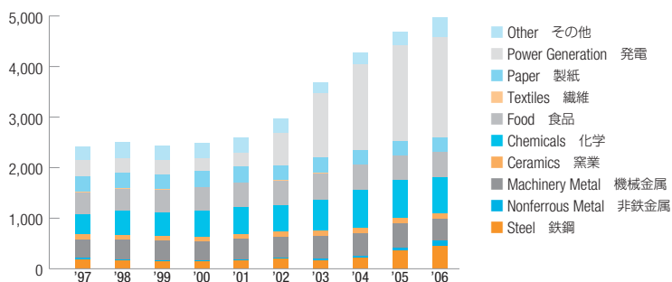
Industrial Use (Million m 3 ) 工業用 (百万m 3 )
