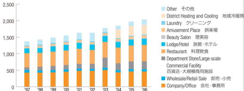
Commercial Use (Million m 3 ) 商業用 (百万m 3 )
