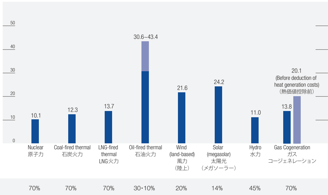
Generation Costs by Power Source (2014 Model Plants) (Yen/kWh) 各電源の発電コスト(2014年モデルプラント) (円/kWh)
